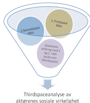
Figur 3. Thirdspace-epistemologisk metodetilnærming.
