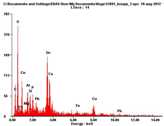
Figur 8 a og b Fnr 10, samankrølla blikkplate med ein 'knopp' i eine enden og sølvgrå flekker på overflata: a) Firkant viser analysert område, b) Resultat av elementanalyse: Kopar (Cu) og bly (Pb) men mest tinn (Sn).
