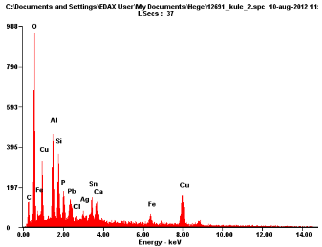
Figur 7 a og b Fnr 10, smelta kule: a) viser analysert område; b) Resultat av elementanalyse: Kopar (Cu), sølv (Ag) og tinn (Sn).
