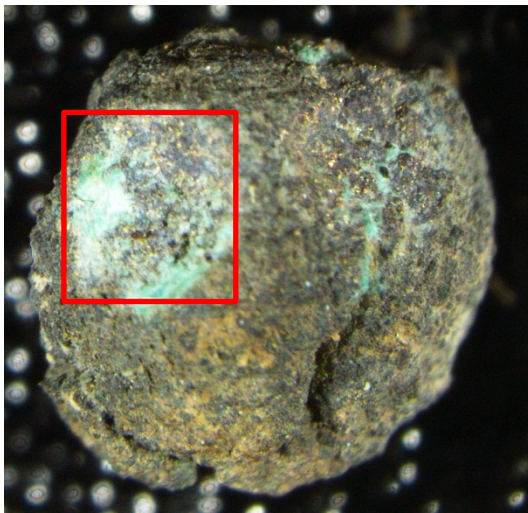
Figur 7 a og b Fnr 10, smelta kule: a) viser analysert område; b) Resultat av elementanalyse: Kopar (Cu), sølv (Ag) og tinn (Sn).
