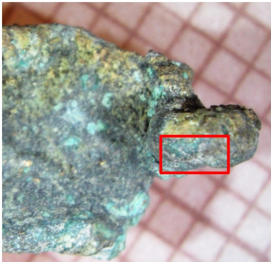
Figur 8 a og b Fnr 10, samankrølla blikkplate med ein 'knopp' i eine enden og sølvgrå flekker på overflata: a) Firkant viser analysert område, b) Resultat av elementanalyse: Kopar (Cu) og bly (Pb) men mest tinn (Sn).
