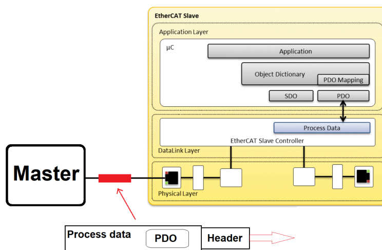
Figur 2.13: PDO kommunikasjon fra master til slave (ref:[25], s.24)
