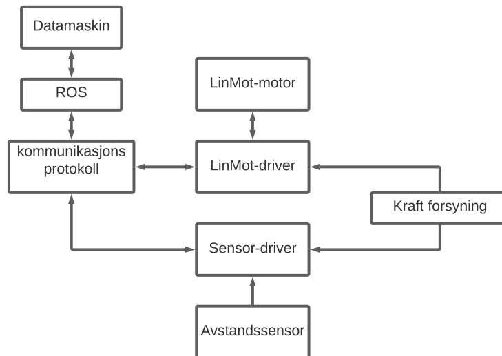
Figur 2.6: Kommunikasjonslinjer i systemet
