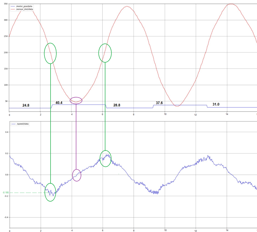
Figur 7.15: Verifisering av posisjonsgraf
