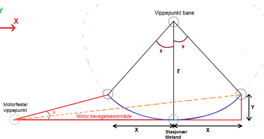
Figur 2.4: Geometrisk sammenheng mellom bevegelige ledd
