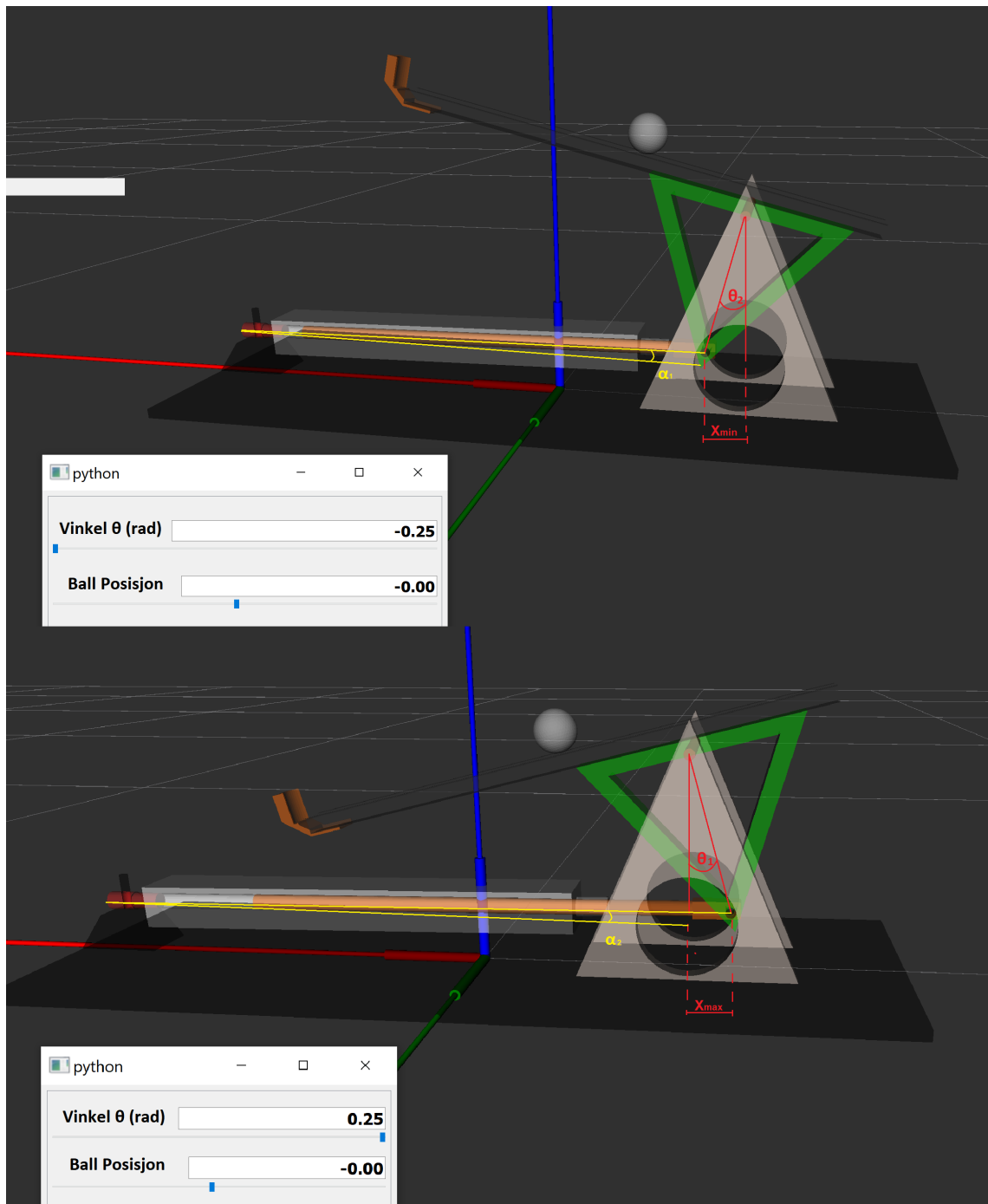
Figur 3.11: Geometrisk sammenheng i RViz
