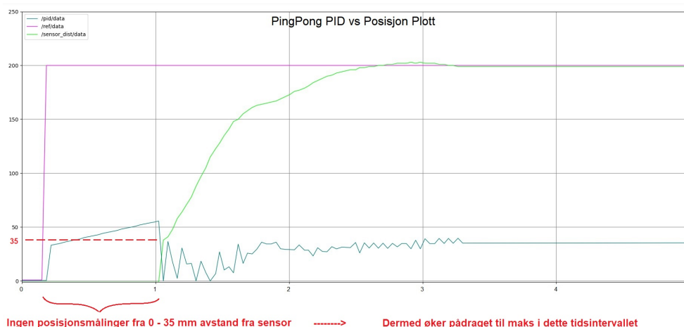
Figur 7.7: Manglende avstandsmålinger i tidsintervall [0, 35] mm
