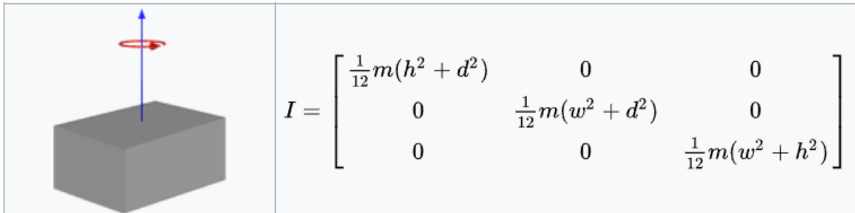
Figur 2.5.1-Treghetsmatrise for kube i rommet [10].
