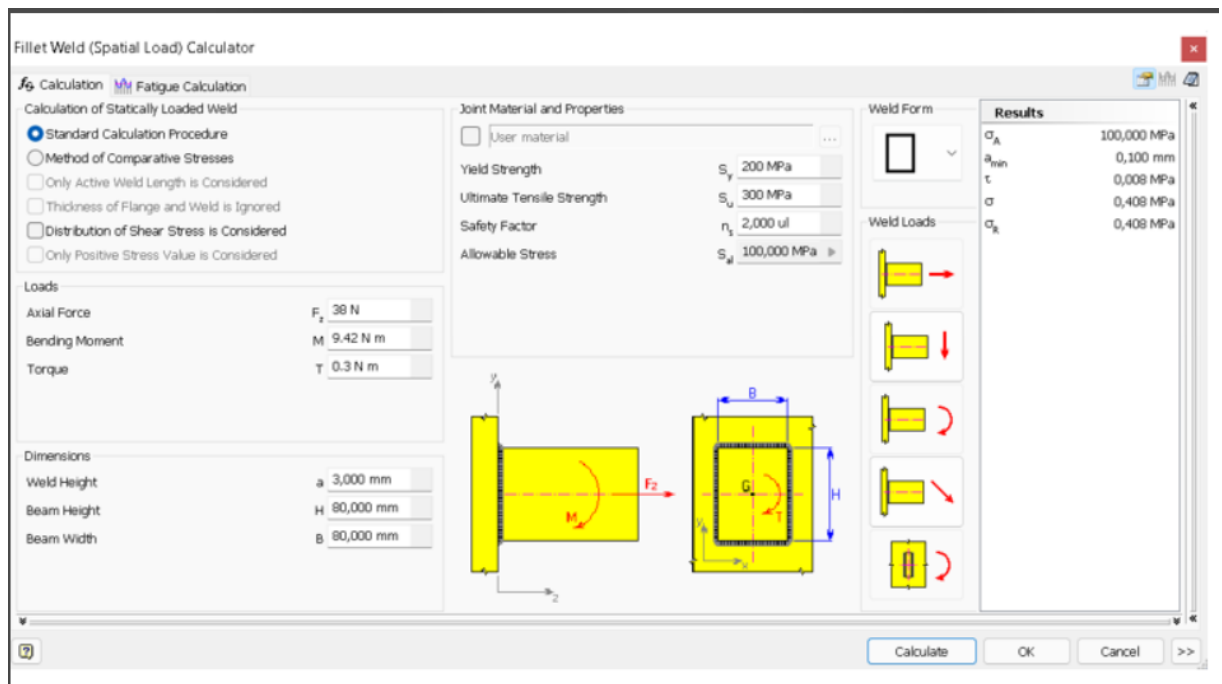
Figur 2.15.1-Eksempel på sveiseberegning i Autodesk Inventor [1].
