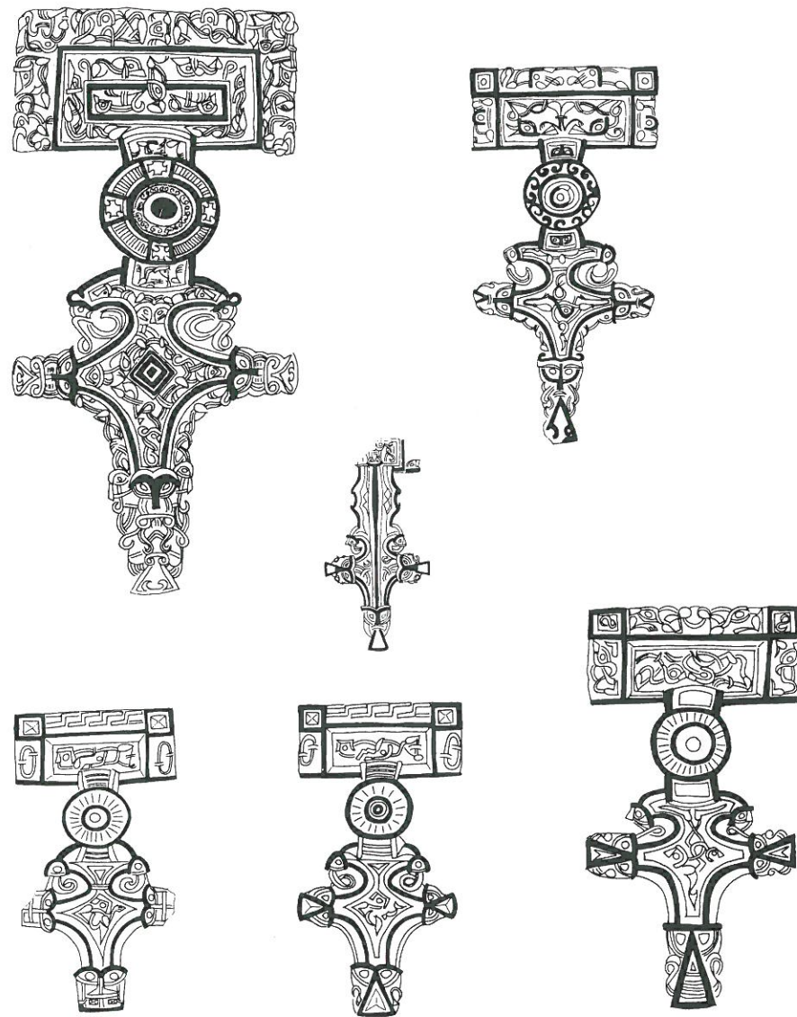
Fig. 8. Relieffspenner i Sognegruppen. Ovenfra, fra venstre: Sandal (F90), Normes (F84), Kvåle (F85), Sørheim (F88), Holum (F83), Syre (F56). Tegning: S.K. 1:2.
