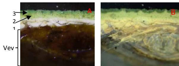
Fig. 48. Detalj av snitt 19 (lerretets malinglag) i pålys (A) og UV (B). Usikkerhet knyttet til antall lag. Har lag 1 stått synlig og er lag 2 og 3 påført samtidig? Er det i så fall en dekor som ikke er fremkommet?
