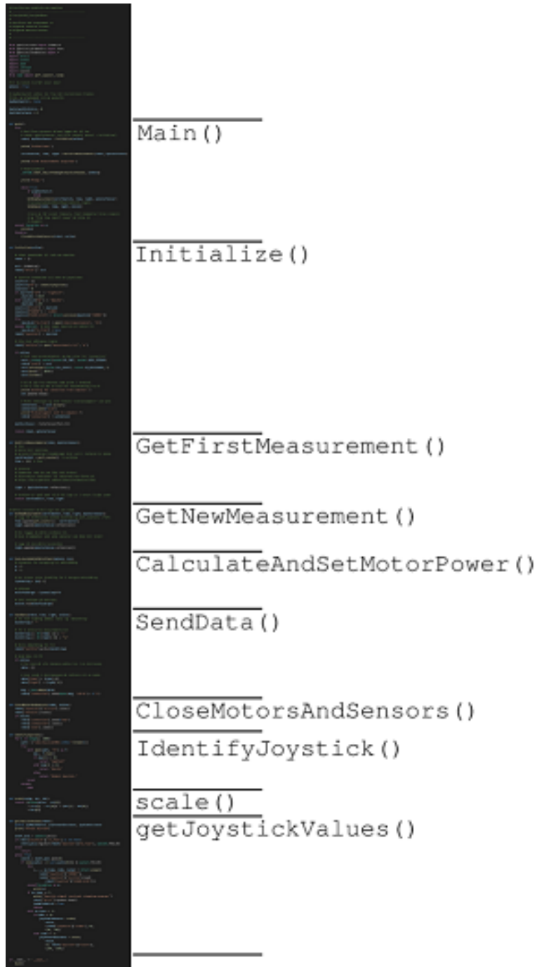
Figur 3.2: Oversikt over koden i EV3main.py.
