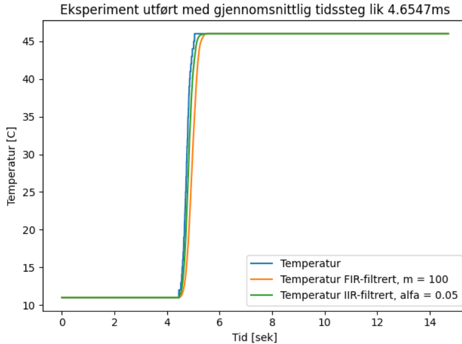
Figur 5.10: Filtrering med m = 100 og \alpha = 0.05 .
