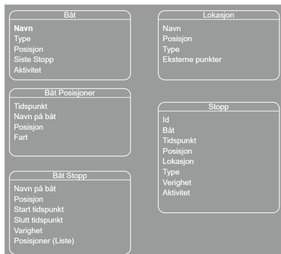
Figur 4.8: Oppbyggingen av database tabellene
