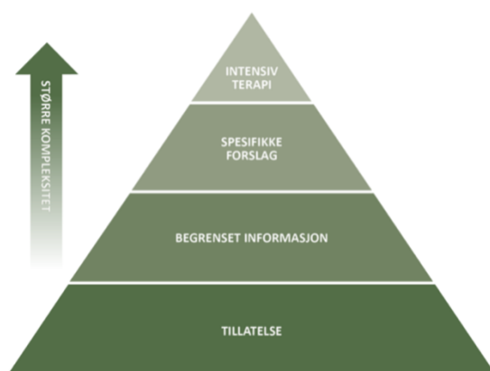
Figur 1. PLISSIT-modellen
